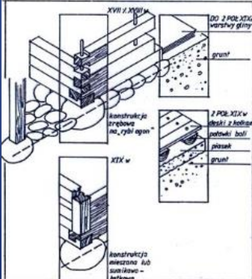
KONSTRUKCJA ŚCIAN, FUNDAMENTOWANIE, WARSTWY PODŁOGI
