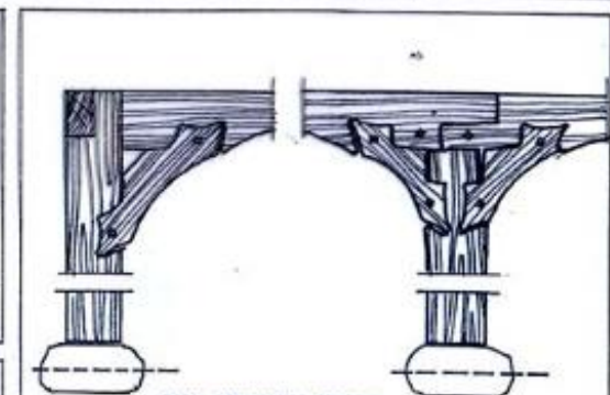
DETAL KONSTRUKCJI PODCIENIA
