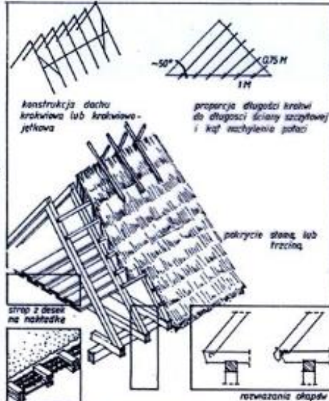
POKRYCIE I KONSTRUKCJA WIEŻBY DACHOWEJ
